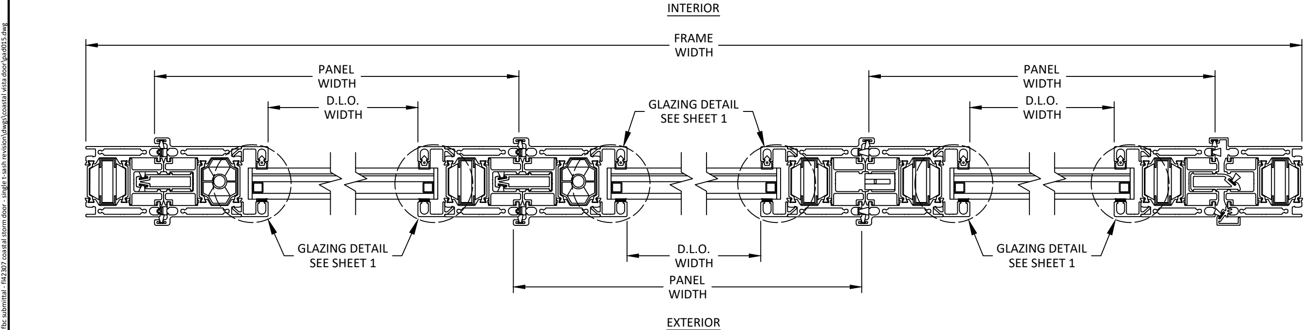
B 5 HORIZONTAL SECTION SLIDING JAMB
